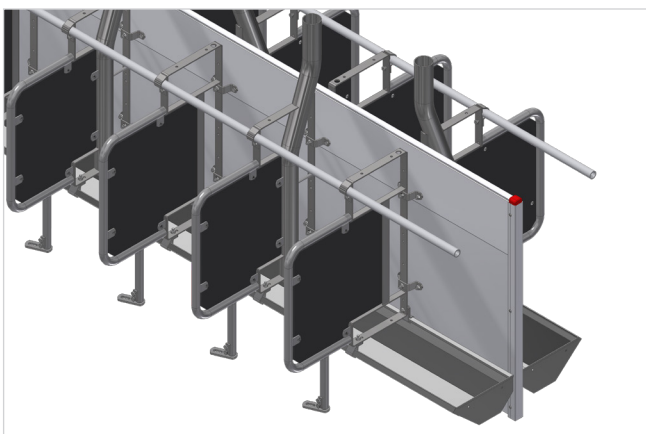
Fressplatzteiler montiert an PVC Brettprofilwand
