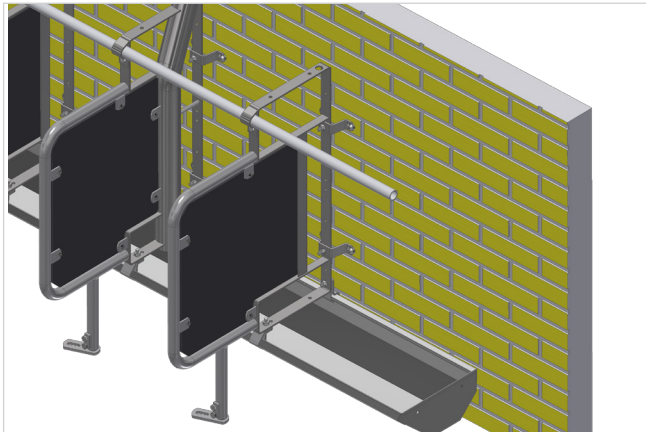
An der Wand montierte Futtertrennwand
