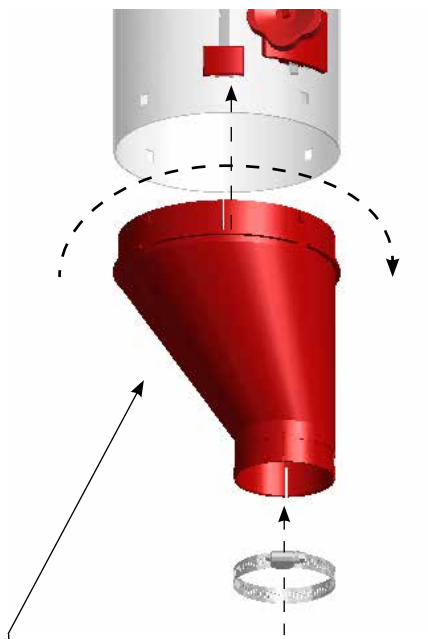
Montage des Trichters "0221-512" Trichter "0221-512" kann in 4 verschiedenen Positionen plziert werden
