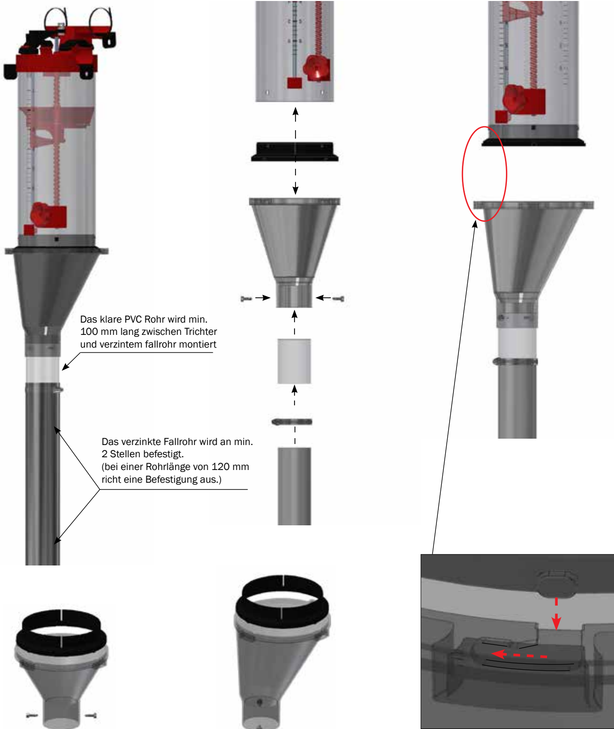
0221-516 VD5 TRICHTER FÜR VD2 ZENTRALER ABGANG
