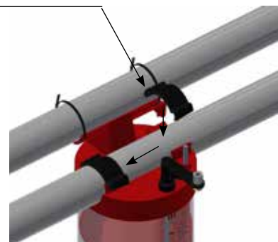
Montage Rohrklammern
