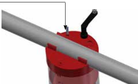
Montage an Ø60mm Rohrleitung
