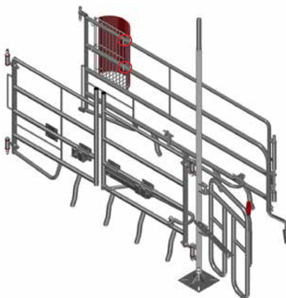
Strohhalter am Farrow Comfort. Wird an den ersten und zweiten rohren in der trennwand montiert. Kann alternativ auch an den zweiten und vierten rohren montiert werden. Er wird an einer festen trennwand ohne öffnungsfunktion installiert.
