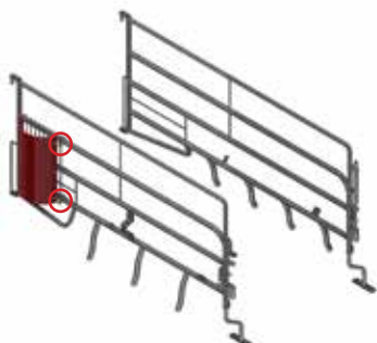
Strohhalter am Welsafe-abferkelstall. Wird an den ersten und zweiten rohren in der trennwand montiert. Kann alternativ auch an den zweiten und vierten rohren montiert werden. Beidseitige montage möglich.
