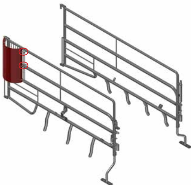
Strohhalter am Welsafe-abferkelstall. Wird an den ersten und zweiten rohren in der trennwand montiert. Kann alternativ auch an den zweiten und vierten rohren montiert werden. Beidseitige montage möglich.
